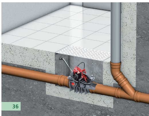
Funktionsweise einer Rückstauklappe 35
